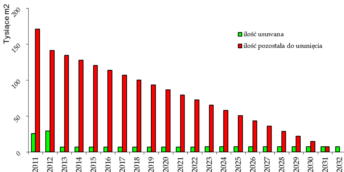
Wykres 7: Proces C – roczne poziomy usuwania określone na podstawie wytycznych z POKzA 2009 – 2032
